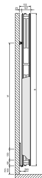
DimensionalDrawing - Kos V / Faro V, tipas 22, vaizdas iš šono
