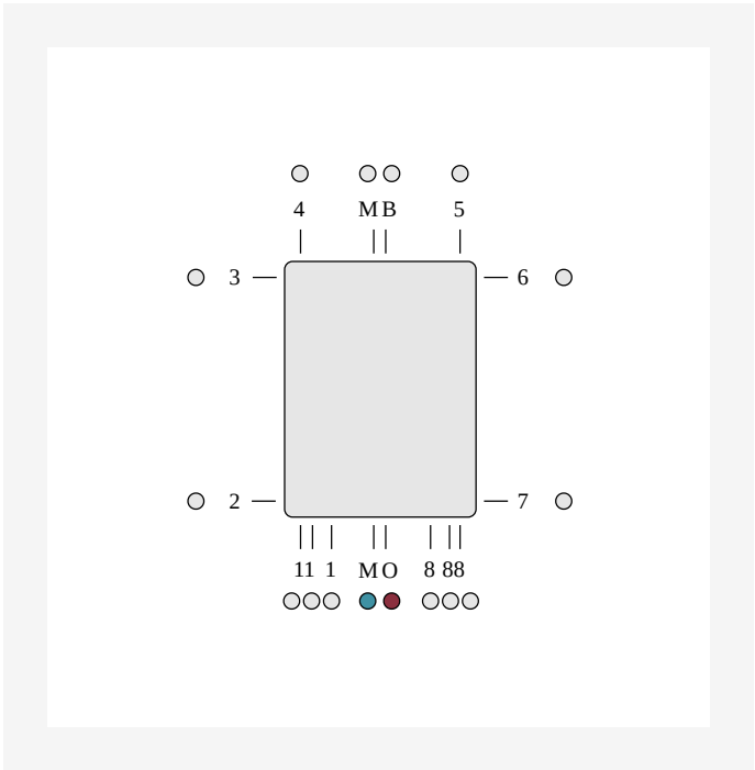
DimensionalDrawing - ETIM OM, vertikali centrinė jungtis
