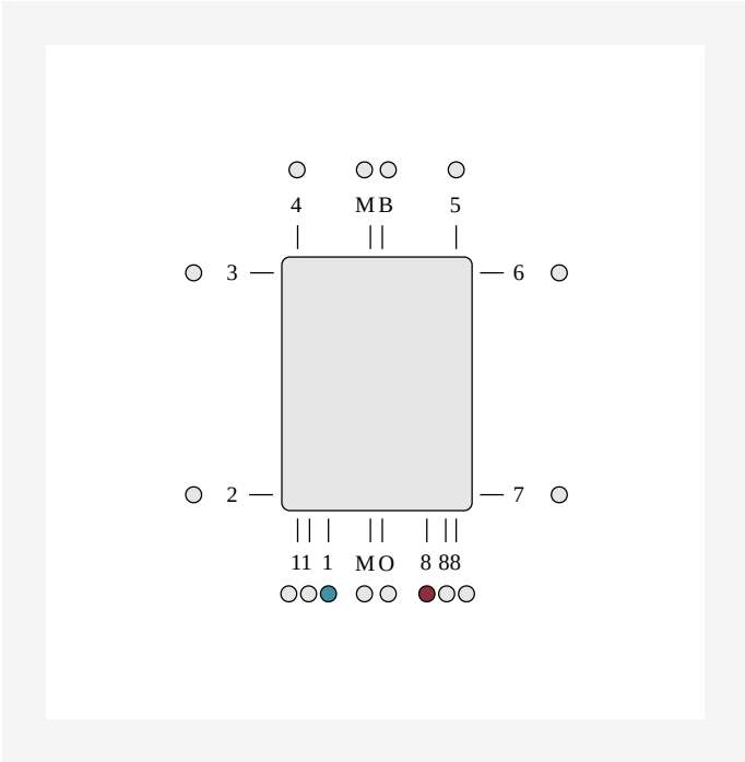
DimensionalDrawing - ETIM 81, vertikali jungtis
