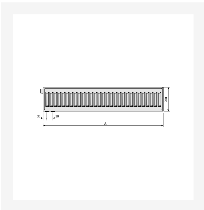
DimensionalDrawing - Plint, Plint P un Plint R, skats no aizmugures
