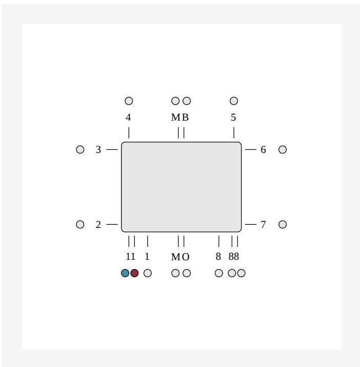
DimensionalDrawing - ETIM 11 apakšējais pieslēgums, ieeja pa labi, izeja pa kreisi. Apakšējais pieslēgums ar integrētu kapilāro cauruli prasa vārsta ieliktna izmantošanu. Neizmantotie pieslēgumi ir aizvērti.
