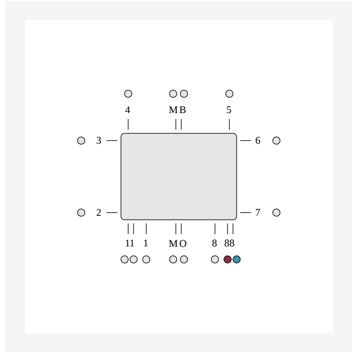
DimensionalDrawing - ETIM 88 LR apakšējais pieslēgums. Apakšējais pieslēgums ar integrētu vārsta prasa vārsta ieliktna izmantošanu. Neizmantotie pieslēgumi ir noslēgti.
