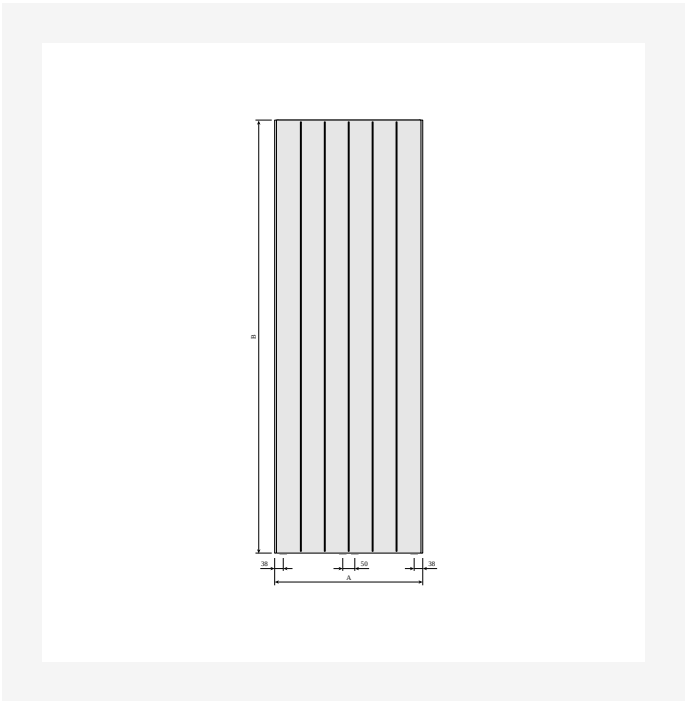
DimensionalDrawing - Faro V, skats no priekšpusē
