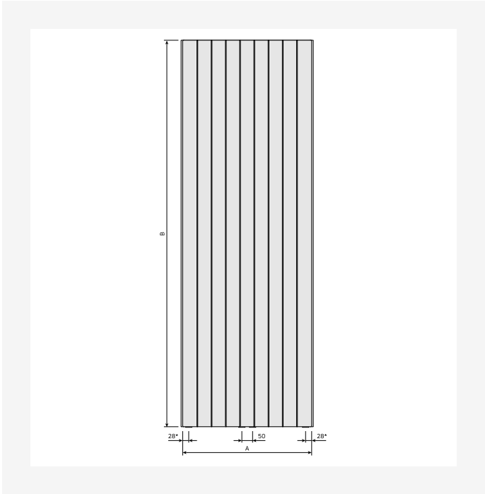
DimensionalDrawing - Faro V, skats no priekšpuses
