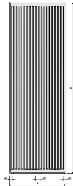
DimensionalDrawing - Vertical ab 2024 Frontansicht Typ 10
