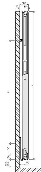
DimensionalDrawing - Vertical ab 2024 Seitenansicht Typ 21
