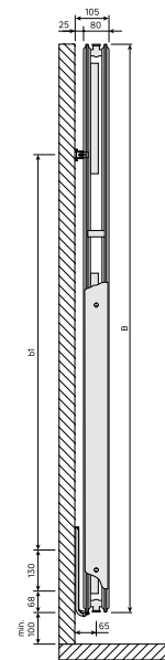
DimensionalDrawing - Vertical ab 2024 Seitenansicht Typ 21
