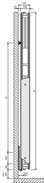
DimensionalDrawing - Vertical ab 2024 Seitenansicht Typ 22
