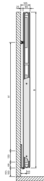
DimensionalDrawing - Vertical ab 2024 Seitenansicht Typ 21
