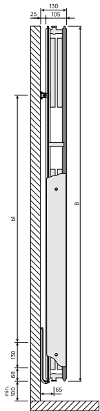
DimensionalDrawing - Vertical ab 2024 Seitenansicht Typ 22
