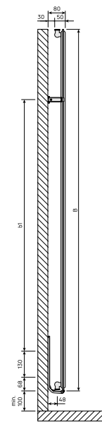
DimensionalDrawing - Vertical ab 2024 Seitenansicht Typ 10
