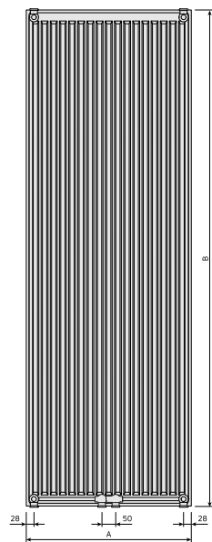
DimensionalDrawing - Vertical ab 2024 Rückansicht Typ 10
