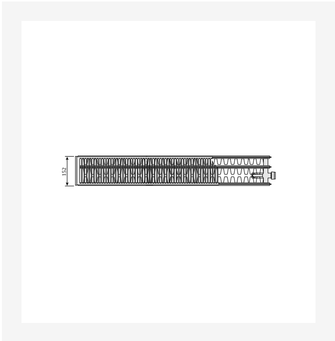
DimensionalDrawing - Ventil Compact Typ 33, Draufsicht, Heizkörper gedreht
