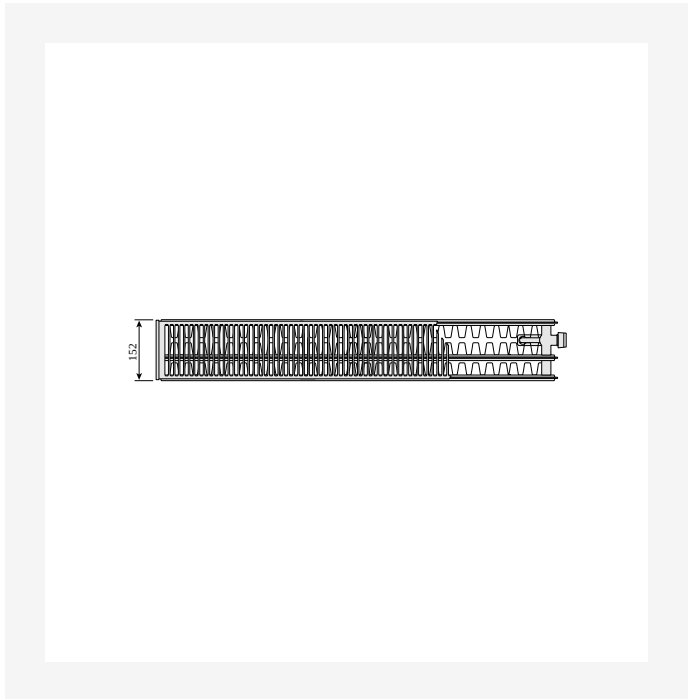
DimensionalDrawing - Ventil Compact Typ 33, Draufsicht
