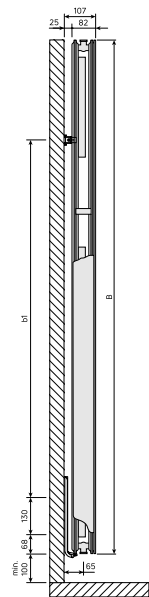
DimensionalDrawing - Kos V / Faro V 2024, Seitenansicht Typ 21
