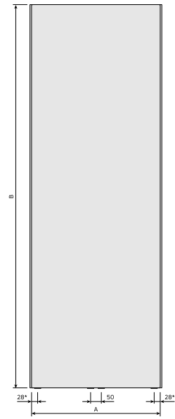
DimensionalDrawing - Kos V 2024 Frontansicht
