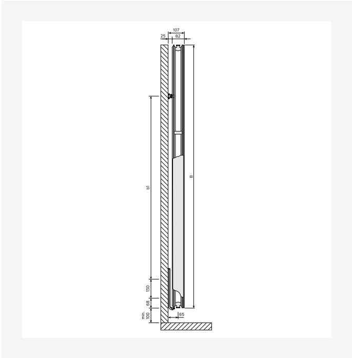
DimensionalDrawing - Kos V / Faro V 2024, Seitenansicht Typ 20
