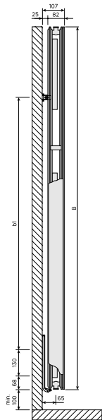
DimensionalDrawing - Kos V / Faro V 2024, Seitenansicht Typ 21
