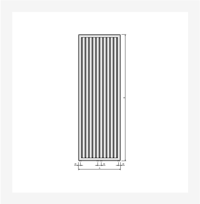
DimensionalDrawing - Vertical type 10, Vue de face - sans joux latérales
