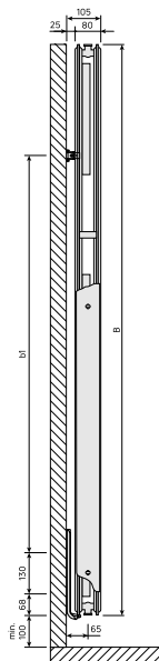
DimensionalDrawing - New_Vertical Vue latérale
