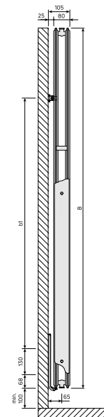
DimensionalDrawing - New_Vertical Vue latérale
