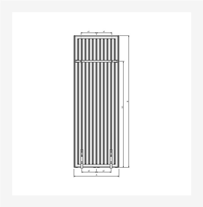
DimensionalDrawing - Vertical avec fixations MCW6, Vue arrière
