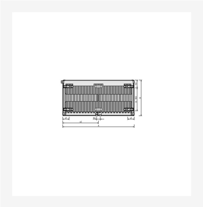
DimensionalDrawing - T6 3010 type 11, Vue arrière
