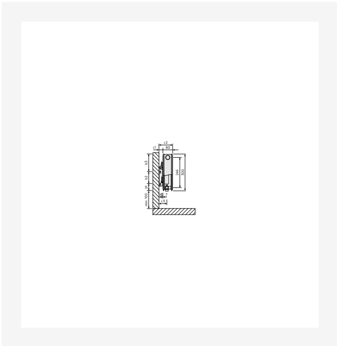
DimensionalDrawing - T6 3010, type 21, Vue de côté
