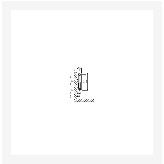
DimensionalDrawing - T6 3010, type 11, Vue de côté
