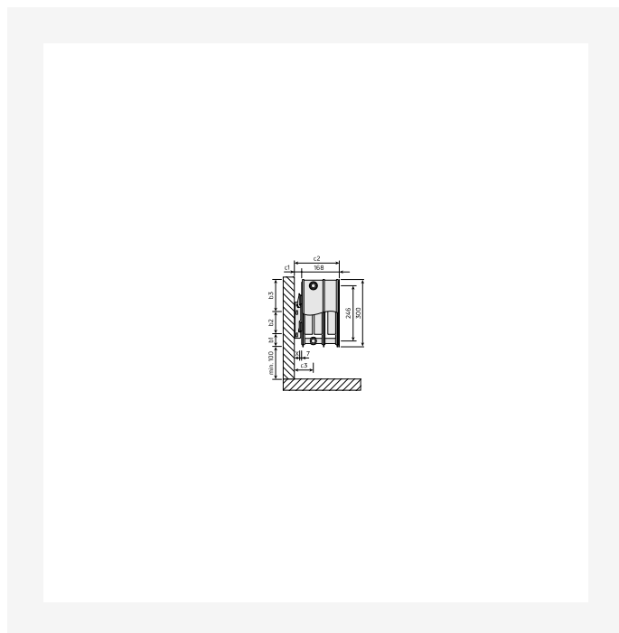
DimensionalDrawing - Reggane 3010 Plan/Deco, type 33 H300, Vue latérale
