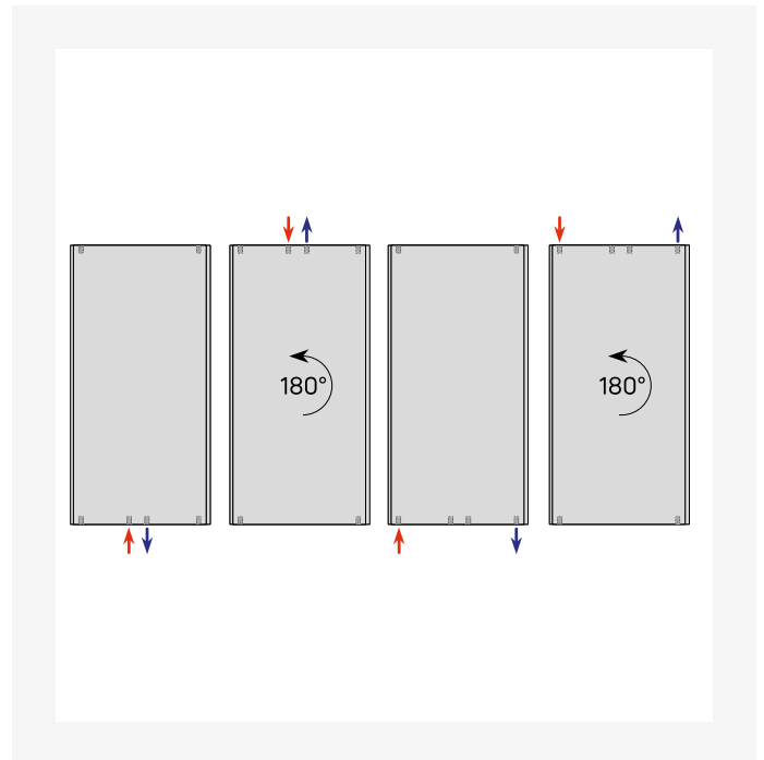
DimensionalDrawing - Pystysuuntaiset liitännävaihtoehdot
