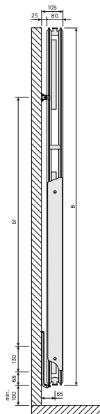
DimensionalDrawing - Vertical, tyyppi 21, sivunäkymä
