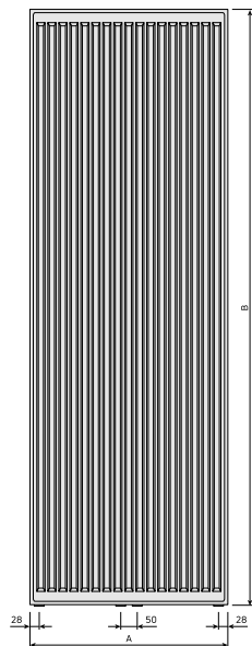
DimensionalDrawing - Vertical, tyyppi 10, etunäkymä
