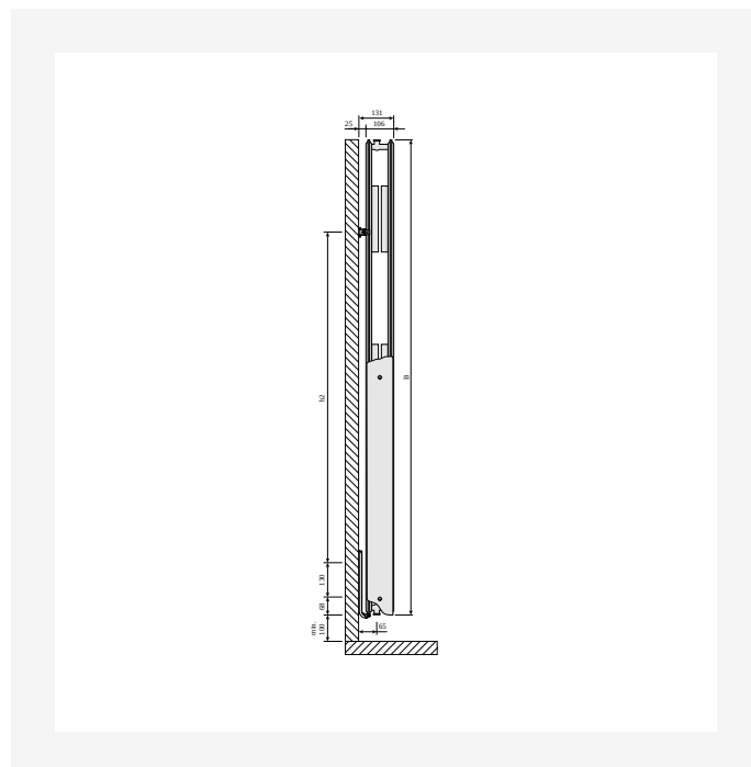
DimensionalDrawing - Vertical, tyyppi 22, sivunäkymä
