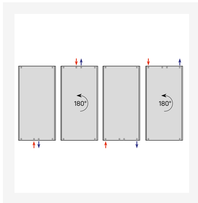
DimensionalDrawing - Pystysuuntaiset liitävaihtoehdot
