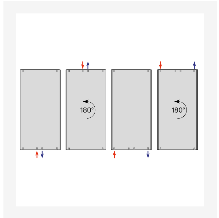
DimensionalDrawing - Pystysuuntaiset liitävaihtoehdot
