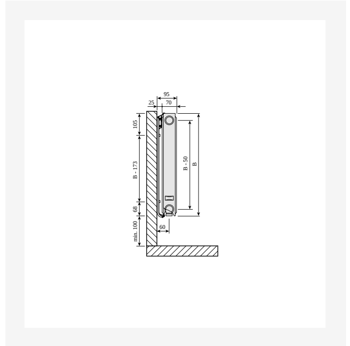
Dimensional Drawing - Ventil Compact, tyyppi 21S, sivulta katsottuna Monclac-kiinnikkeillä
