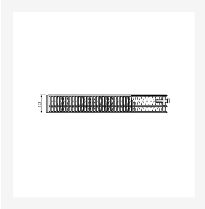
Dimensional Drawing - Ventil Compact, tyyppi 33, ylhäältä katsottuna
