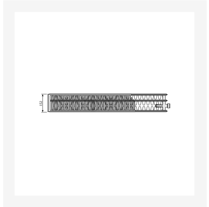
Dimensional Drawing - Ventil Compact, tyyppi 33, ylhäältä katsottuna
