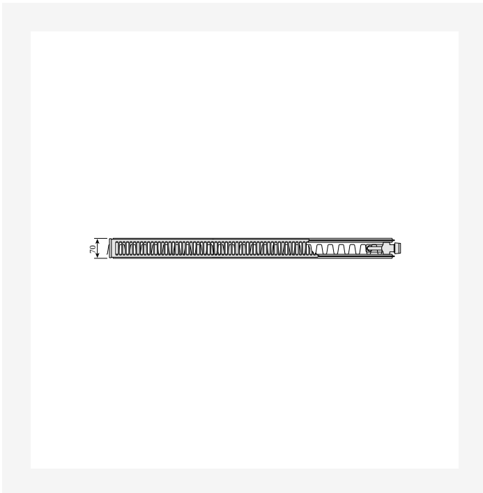
Dimensional Drawing - Ventil Compact, tyyppi 21S, ylhäältä katsottuna
