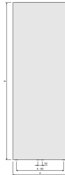
DimensionalDrawing - Tinos V, etunäkymä
