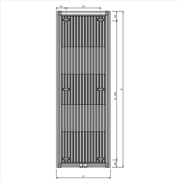
DimensionalDrawing - Tinos V, tyyppi 11, takaa
