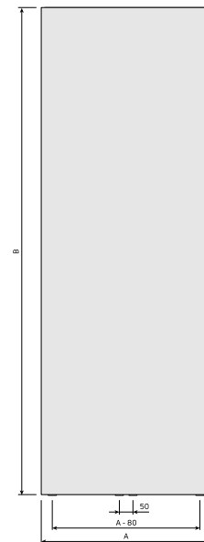
DimensionalDrawing - Tinos V, etunäkymä
