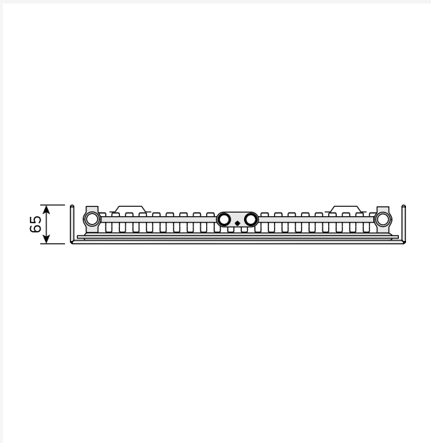
DimensionalDrawing - Tinos V, tyyppi 11, ylhäältäpäin
