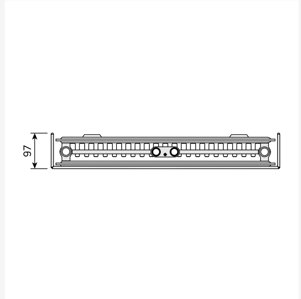
DimensionalDrawing - Tinos V, tyyppi 21, ylhäältäpäin
