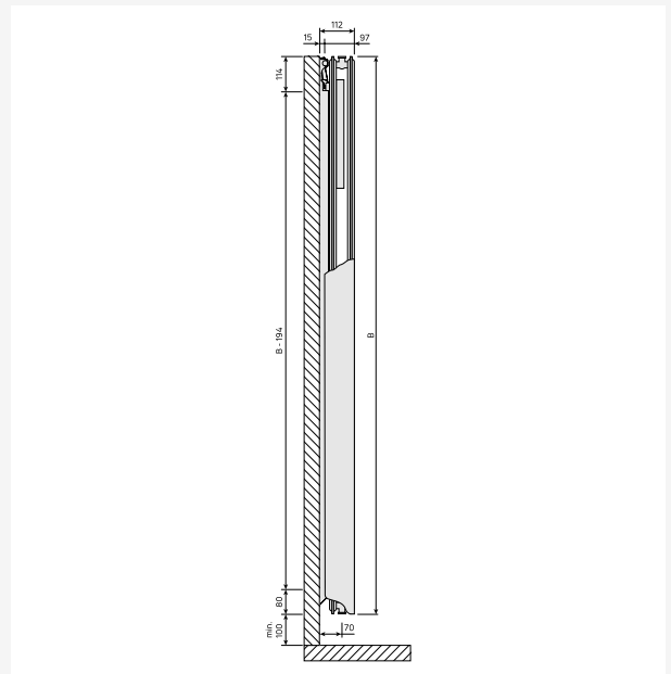
DimensionalDrawing - Tinos V / Paros V, tyyppi 21, sivunäkymä
