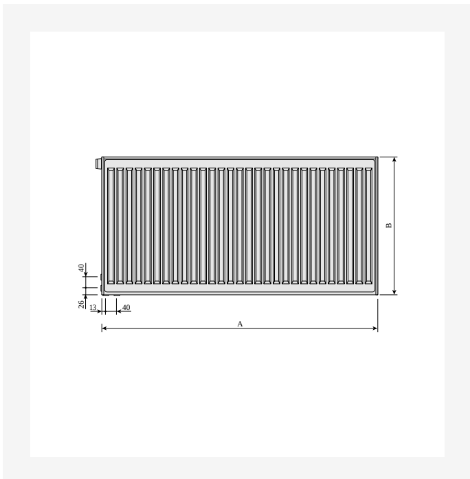
DimensionalDrawing - Thermopanel, etunäkymä, vasen
