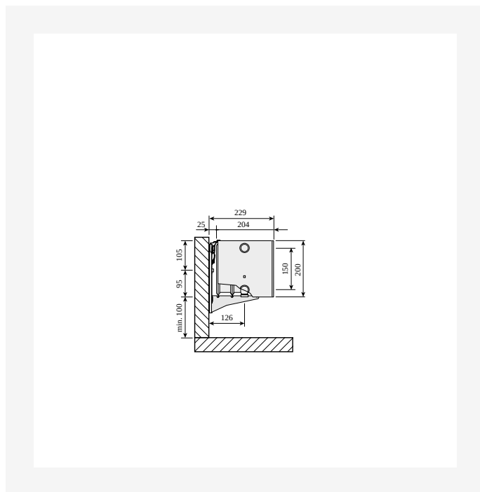
DimensionalDrawing - Plint P ja Plint R, tyyppi 44, sivunäkymä Monclac-seinäkannakkeilla
