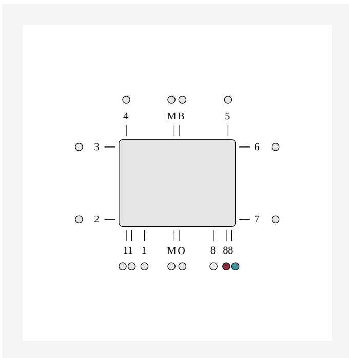
DimensionalDrawing - ETIM 88 LR alaliitäntä. Integroitu venttiili vaatii venttiilisisäkkeen käytön. Käyttämättömät liitännät on tulpattu.
