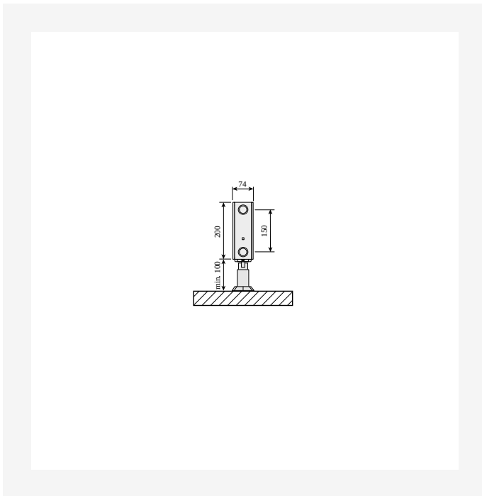
DimensionalDrawing - Plint PD ja Plint RD, tyyppi 21s, lattiatalineillä, sivunäkymä
