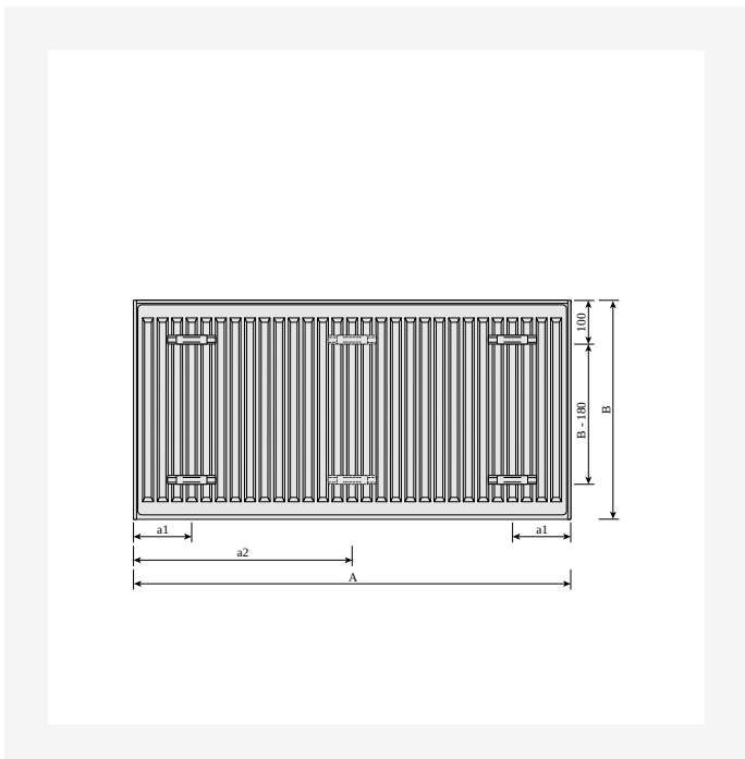
DimensionalDrawing - Plan Compact, takanäkymä
