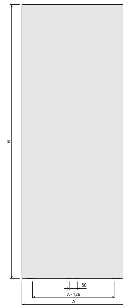
DimensionalDrawing - Paros V, tyyppi 11, etunäkymä
