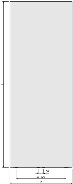
DimensionalDrawing - Paros V, tyyppi 11, etunäkymä
