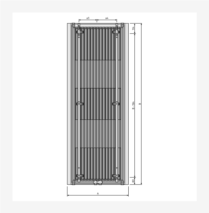
DimensionalDrawing - Paros V, tyyppi 11, takaa MCWV-kannakkeilla
