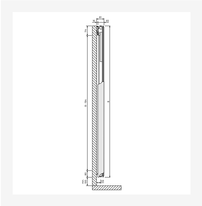
DimensionalDrawing - Tinos V / Paros V, tyyppi 11, sivunäkymä
