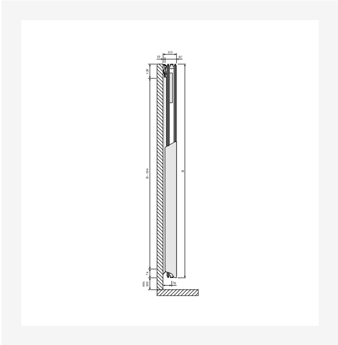
DimensionalDrawing - Tinos V ja Paros V, tyyppi 21, sivunäkymä
