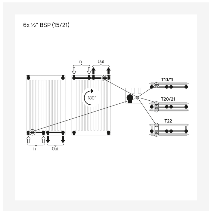
Installation - Myson Plan & Plan Plus Vertical - Liitöntäavaihtoehdot
