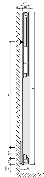
DimensionalDrawing - Kos V / Faro V, tyyppi 21, sivunäkymä
