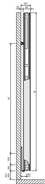
DimensionalDrawing - Kos V / Faro V, tyyppi 21, sivunäkymä
