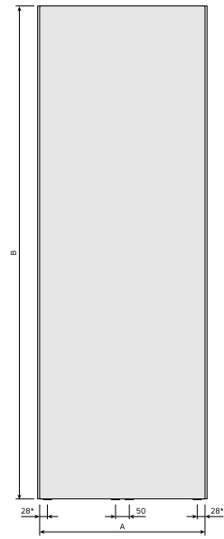
Dimensional Drawing - Kos V, etunäkymä
