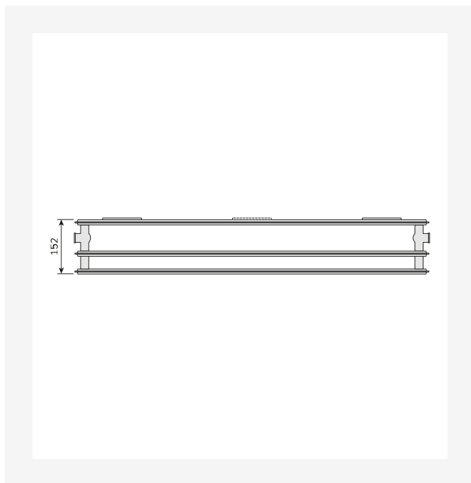
DimensionalDrawing - Hygiene, tyyppi 30, ylhäältäpäin
