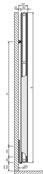
DimensionalDrawing - Kos V / Faro V, tyyppi 20, sivunäkymä
