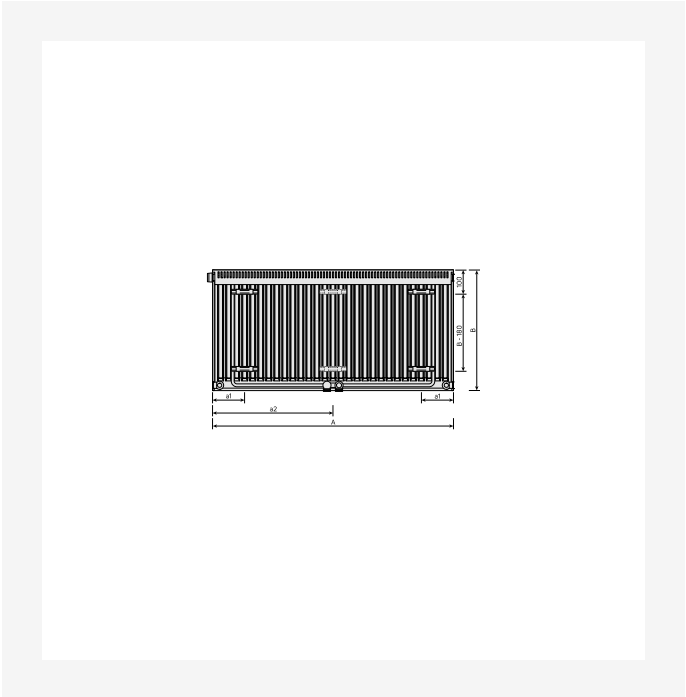
Dimensional Drawing - Flex, tyyppi 11, takaa
