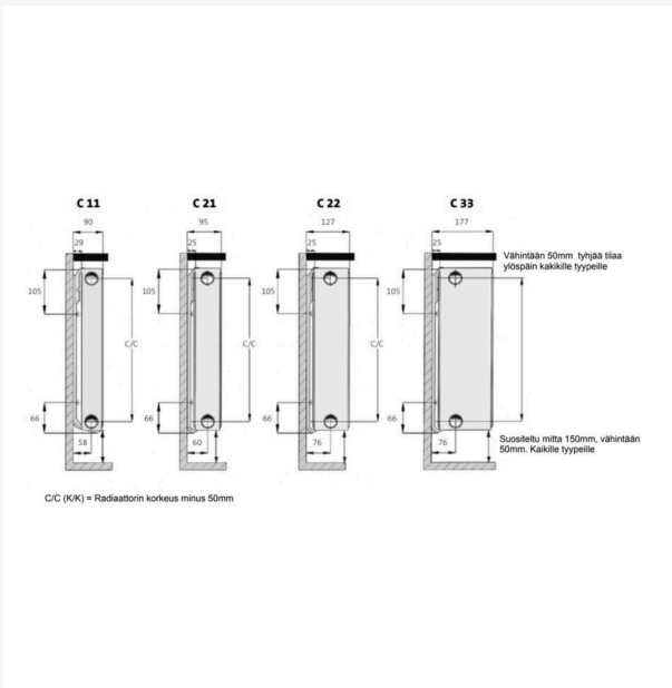
DimensionalDrawing - Radiaattorin kannakointiohje
