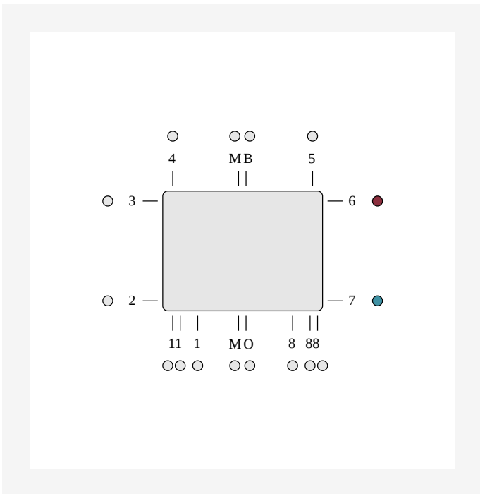
DimensionalDrawing - Sivuliitântä ETIM 67. Sivuliitântä edellyttää ulkoisen patteriliittimen tai venttiilin käyttöä. Sivuliitännän tapauksessa alaosien liitännät tulpataan.
