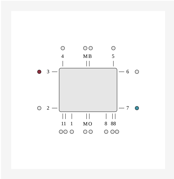
DimensionalDrawing - Diagonaaliliitäntä ETIM 37. Diagonaaliliitäntä edellyttää ulkoisen venttiilin käyttöä. Diagonaaliliitäntännä tapauksessa alaosien liitännät tulpataan.
