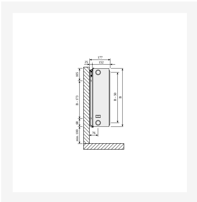
DimensionalDrawing - Compact, tyyppi 33, sivukuva Monclac-seinäkiinnikkeillä
