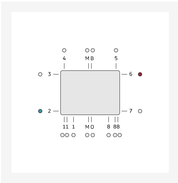
DimensionalDrawing - Diagonaaliliitäntä ETIM 62. Diagonaaliliitäntä edellyttää ulkoisen venttiilin käyttöä. Diagonaaliliitäntännä tapauksessa alaosien liitännät tulpataan.
