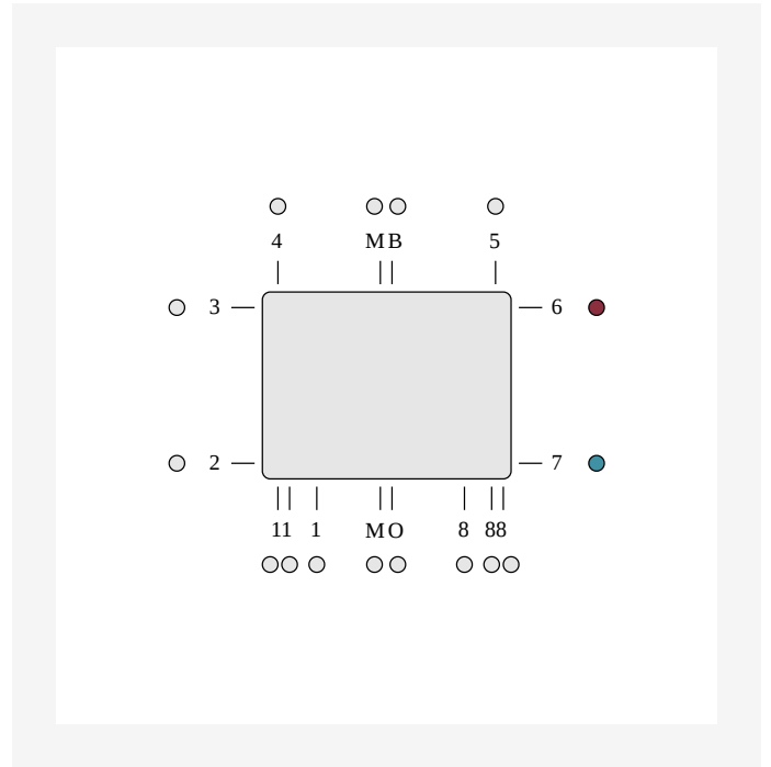
DimensionalDrawing - Sivuliitäntä ETIM 67. Sivuliitäntä edellyttää ulkoisen patteriliittimen tai venttiilin käyttöä. Sivuliitäntännä tapauksessa alaosien liitännät tulpataan.
