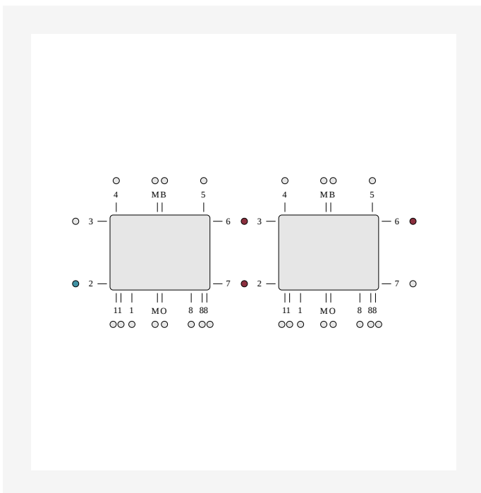
DimensionalDrawing - ETIM 62 Sarjaankytcentä vaakasuora liittäntä
