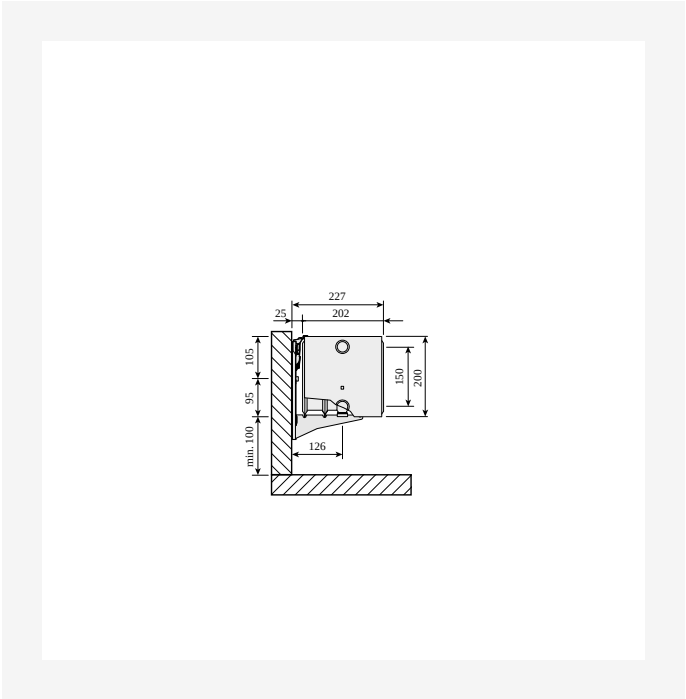
DimensionalDrawing - Plint, tüüp 44, külgsuurt vaade Monclac seinakanduritega
