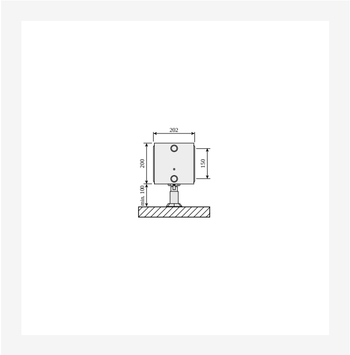
DimensionalDrawing - Plint, tüüp 44, pörandakinnitustega, külgsuurt vaade
