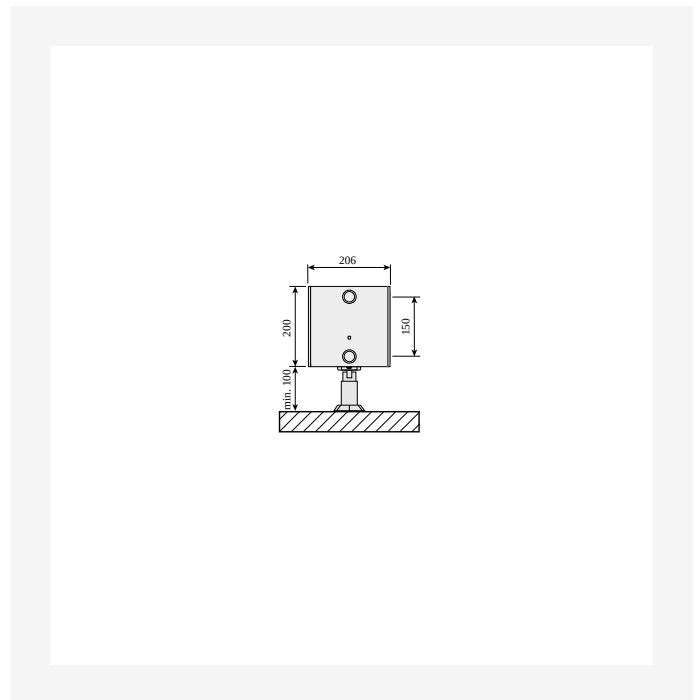
DimensionalDrawing - Plint PD ja Plint RD, tüüp 44, pörandakinnitustega, külgvaade
