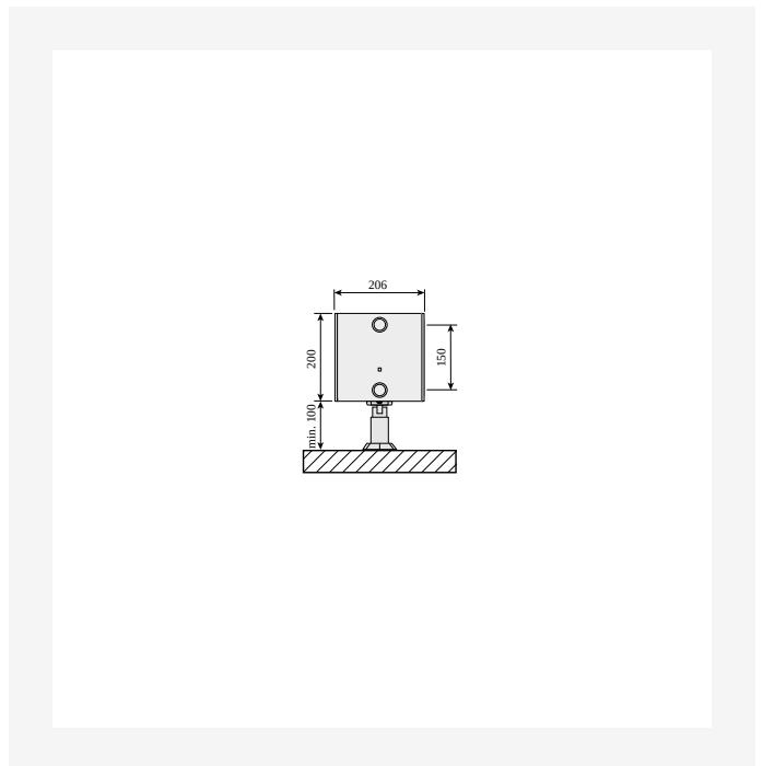
DimensionalDrawing - Plint PD ja Plint RD, tüüp 44, põrandakinnitustega, külgvaade
